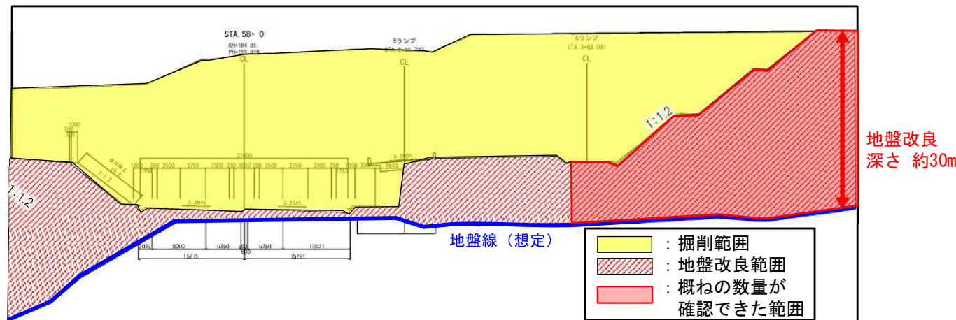
A-A断面
