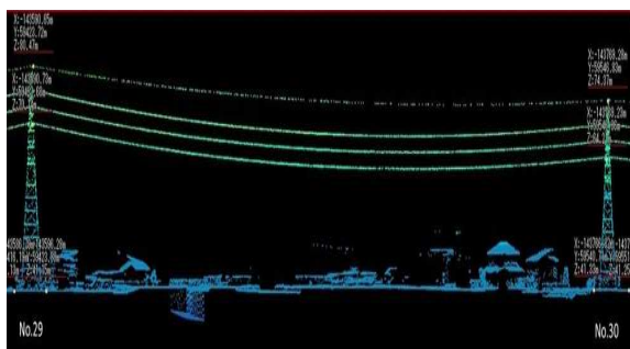
航空レーザ測量により高圧送電線の高さを計測
