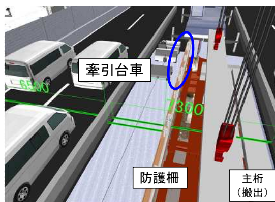
(変更)牽引台車にて搬出
