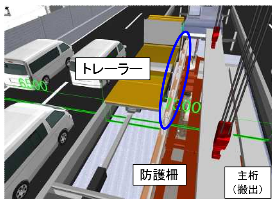
(当初)トレーラーにて搬出
